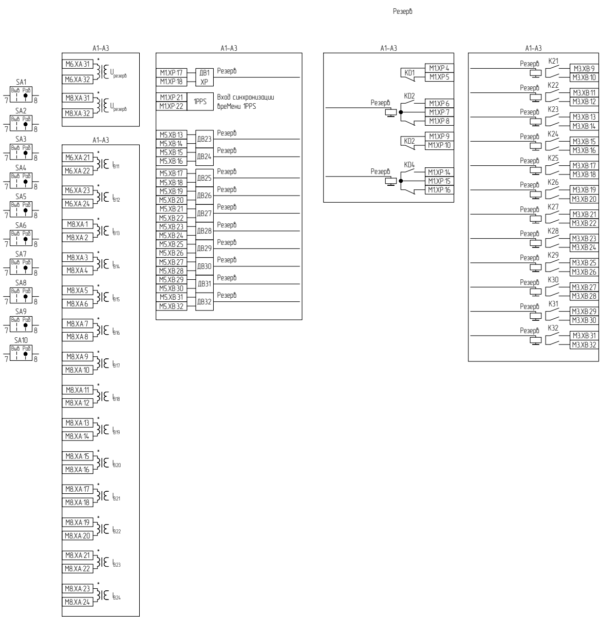
Рисунок В.9 – Схема электрическая принципиальная (часть 9)
