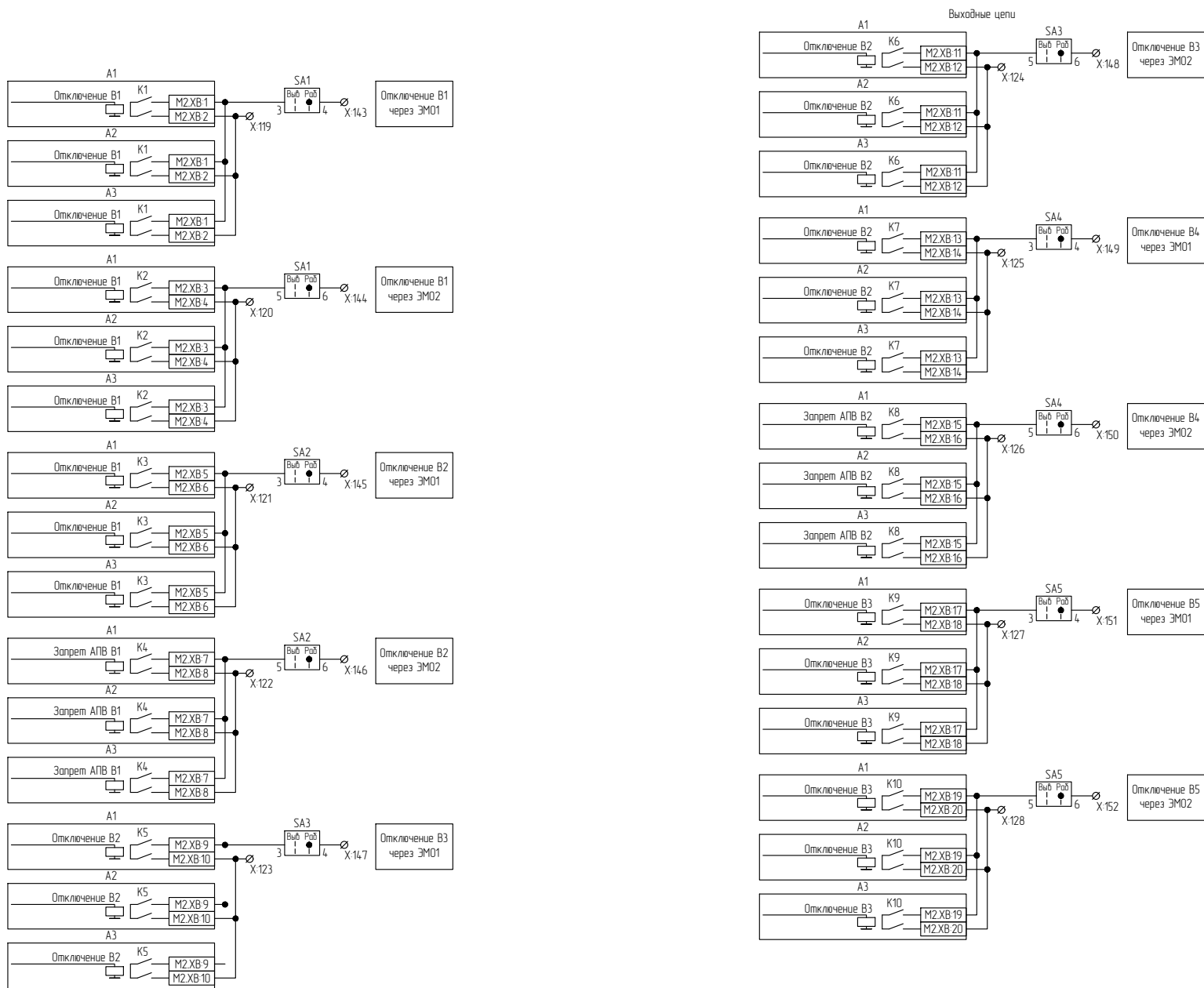
Рисунок В.6 – Схема электрическая принципиальная (часть 6)
