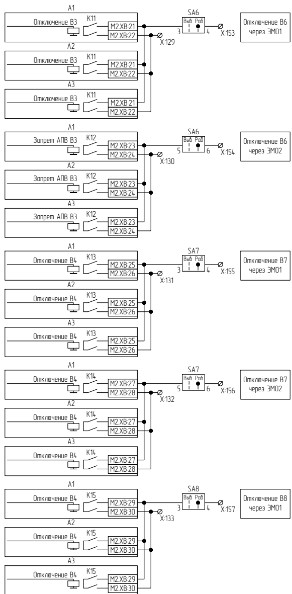
Рисунок В.7 – Схема электрическая принципиальная (часть 7)
